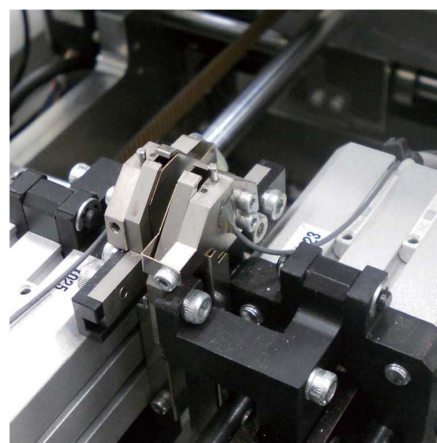
可调 剪脚&amp;弯脚机构
